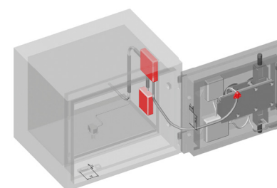
mechaniczny zamek szyfrowy
